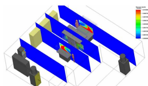
Plans verticaux des concentrations en polluants aux différents postes de travail
